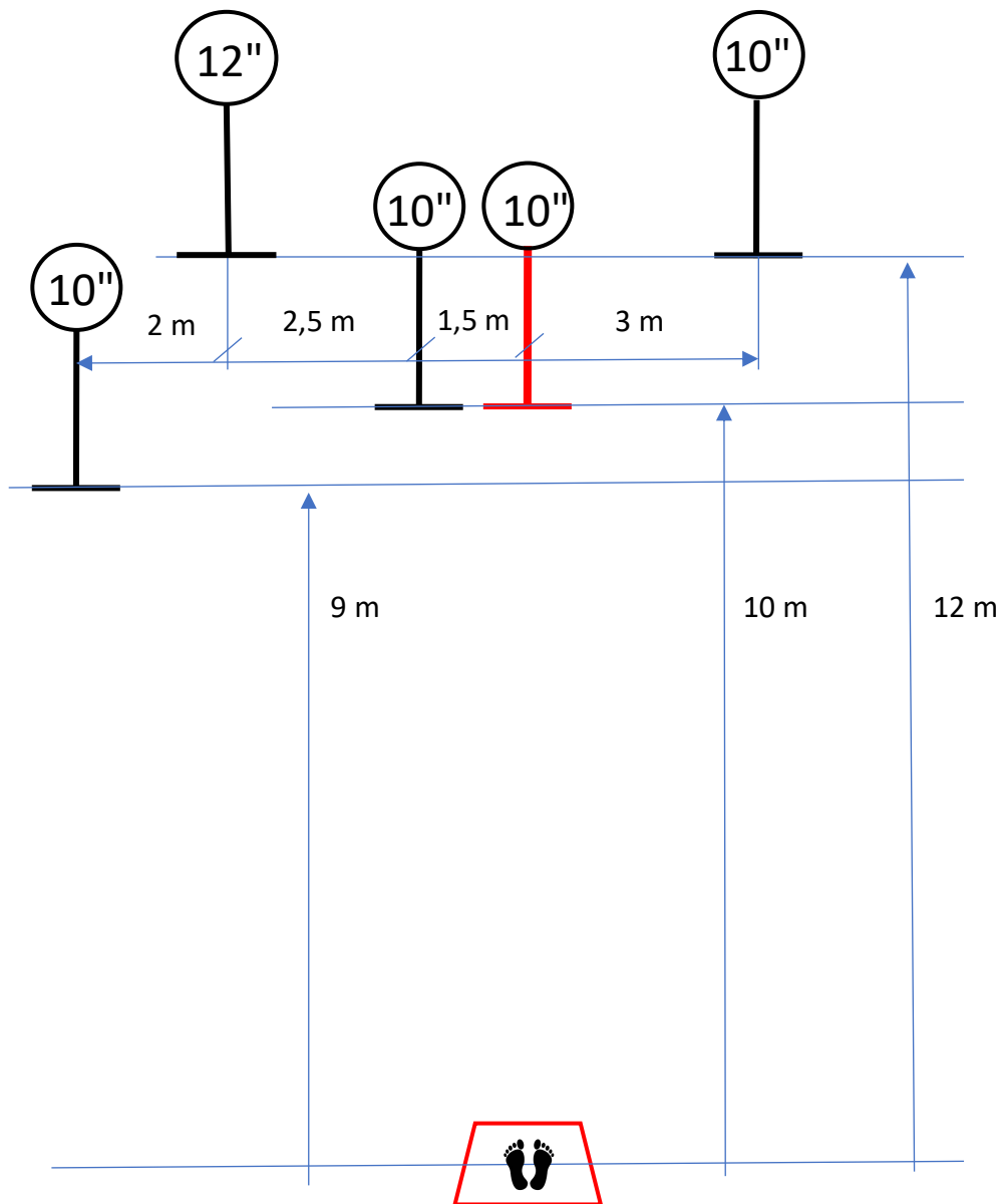
Steel Challenge 1.b pálya
